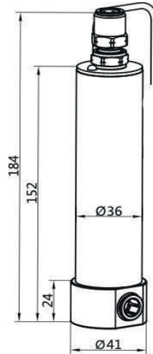
Abbildung 7: Abmessungen Gehäuse
