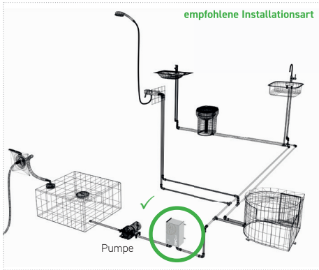
Abbildung 5: Installationsorte
