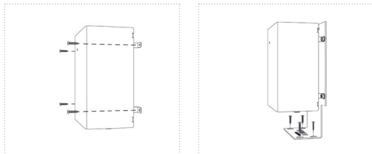
Figure 6 : installation recommandée de l'UV-8 steel sur un mur (raccordement eau IN et OUT orienté vers le bas)
