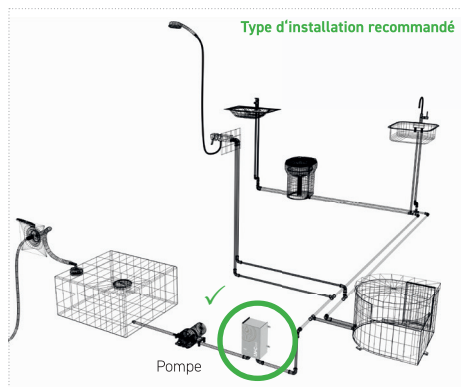
Figure 5 : Lieux d'installation
