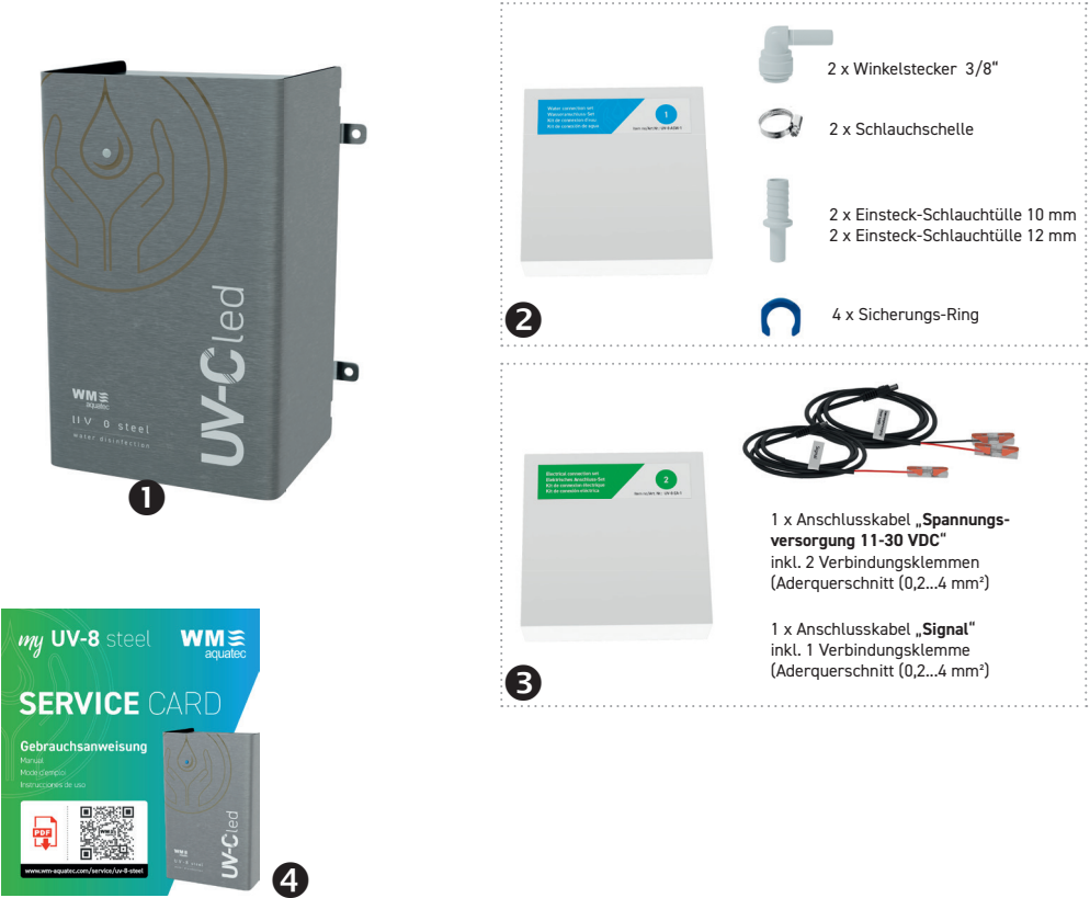
Abbildung 2: Lieferumfang
