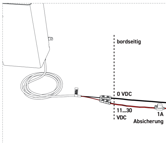
Abbildung 15: Elektrischer Anschluss (Spannungsversorgung)
