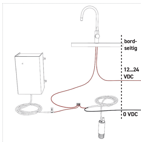
Abbildung 16: Elektrischer Anschluss (Signal) mit Tauchpumpe
