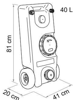
Roll-Tank 40 W
