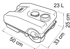
Roll-Tank 23 W
