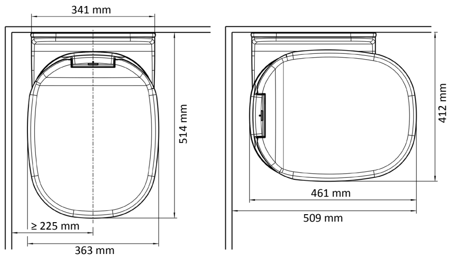
Hauptmaße
