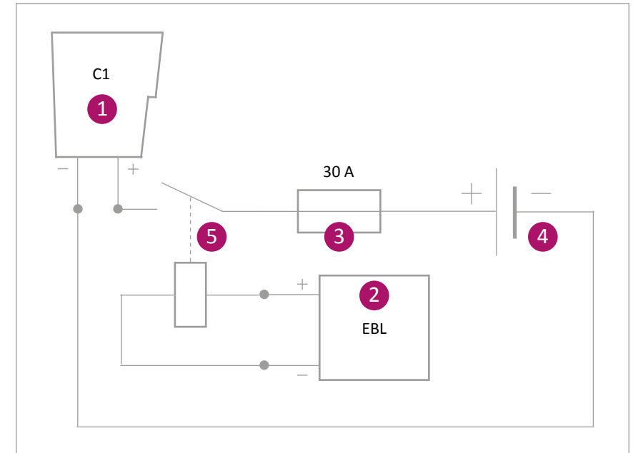
Abb. 2: Anschlussplan Clesana C1
