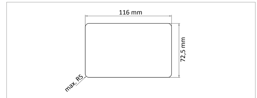
Abb. 7: Erforderliche Maße der Wandöffnung
