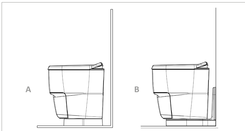
Abb. 1: Einbauort wählen
