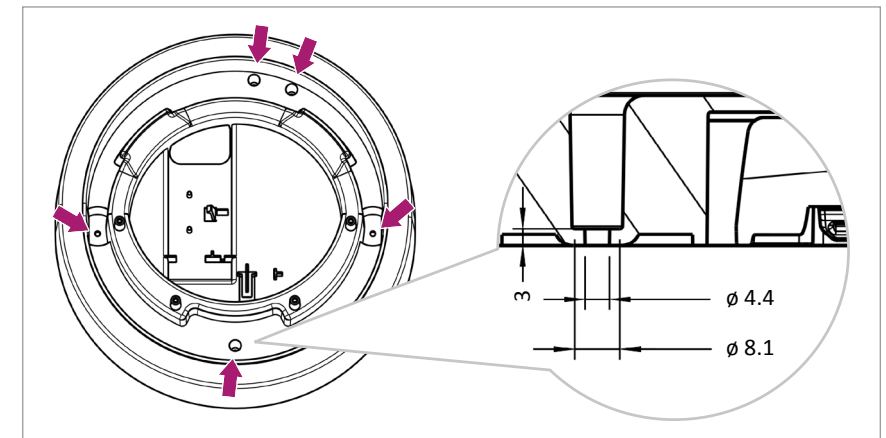
Abb. 5: Montagelöcher für Verschraubung am Boden
