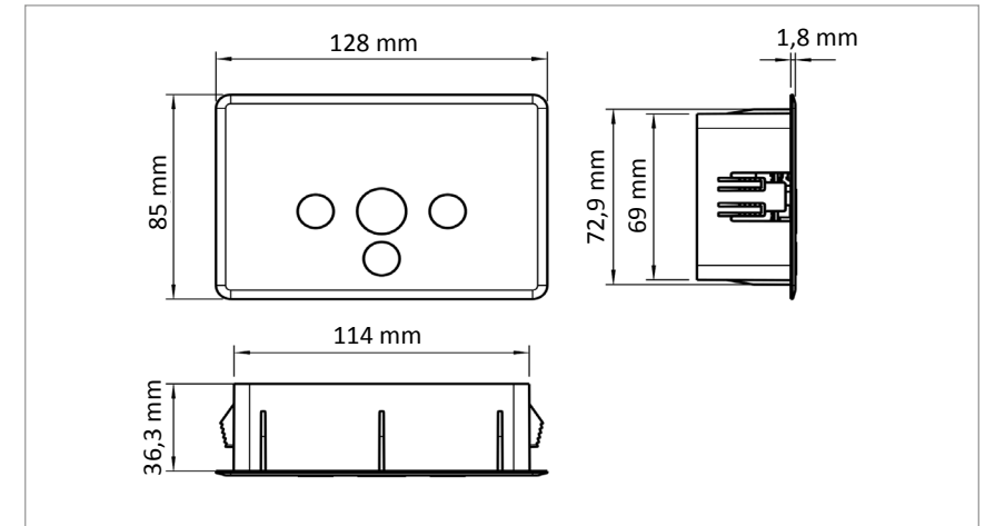
Abb. 6: Abmessungen des Bedienpanels
